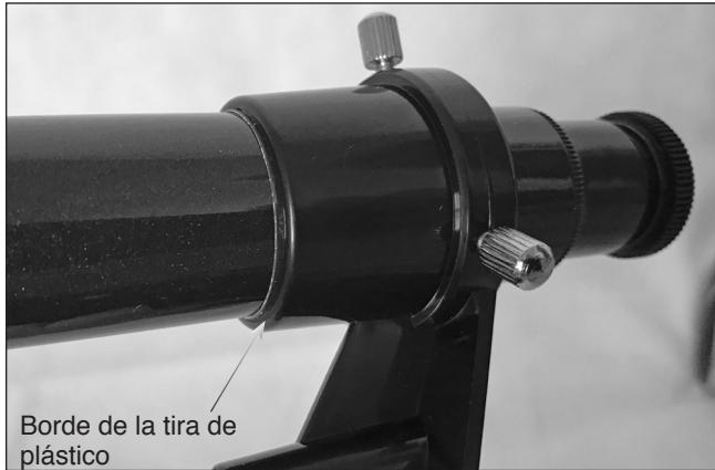
Figura 8. Deslice primero el extremo del ocular del tubo del telescopio buscador, a través del soporte, asegurándose de que la tira de plástico rodea el tubo. La tira apenas debe ser visible cuando el telescopio buscador esté completamente insertado, tal como se indica.
