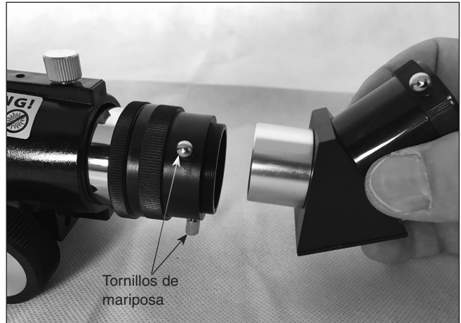
Figura 10. Inserte la diagonal de imagen correcta de 45 grados en el tubo del enfocador y sujétela con los dos tornillos de mariposa.
